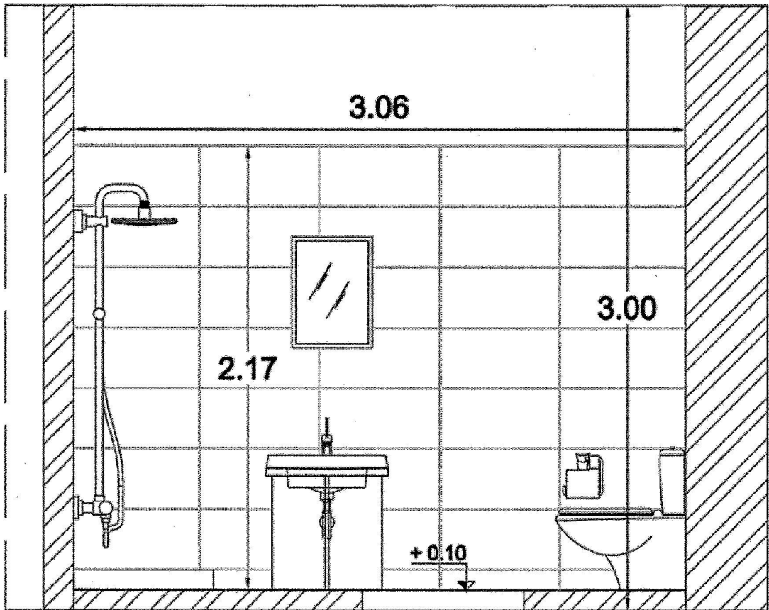
ΤΟΜΗ Α-Α W.C. ΙΑΤΡΕΙΟΥ ΑΝΑΙΣΘΗΣΙΟΛΟΓΙΚΟΥ - 3ος ΟΡΟΦΟΣ_Γ' ΚΤΙΡΙΟ
