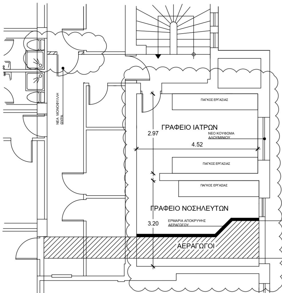
ΚΑΤΟΨΗ ΒΟΗΘΗΤΙΚΩΝ ΧΩΡΩΝ ΠΑΤΑΡΙΟΥ
